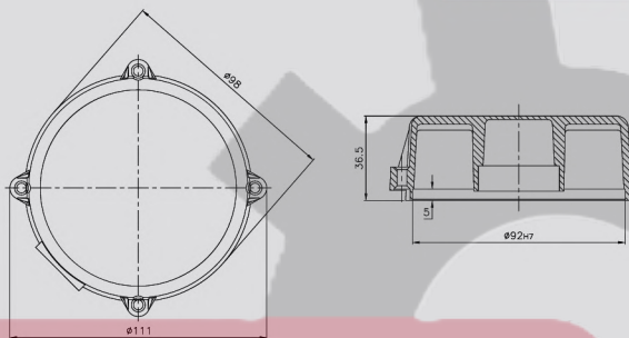
درپوش عقب مشعل گاز سوز سری HA
