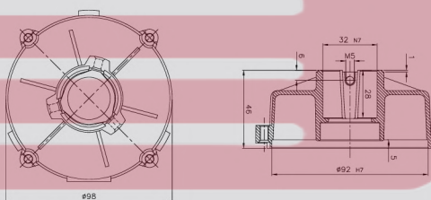
درپوش عقب مشعل گازوئیل سوز سری HA
