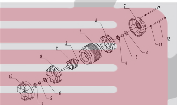
لیست قطعات الکتروموتور هود تک سر شفت و دو سر شفت
